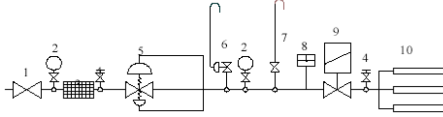
Şekil 32 Atmosferik brülör doğa l gaz kontrol hattı ekipmanları
