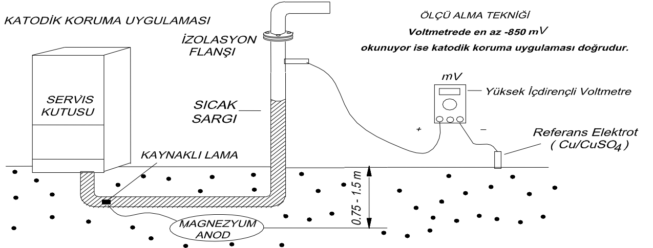
Şekil 5 Katodik Koruma Uygulaması
