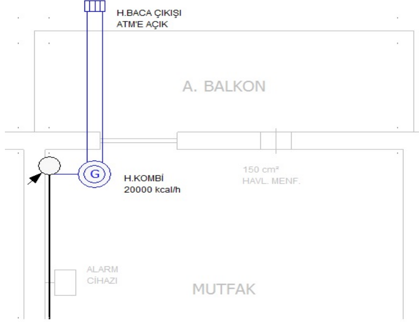
Şekil 23 – Cihaz bacalarının balkon dışına uzatılması
