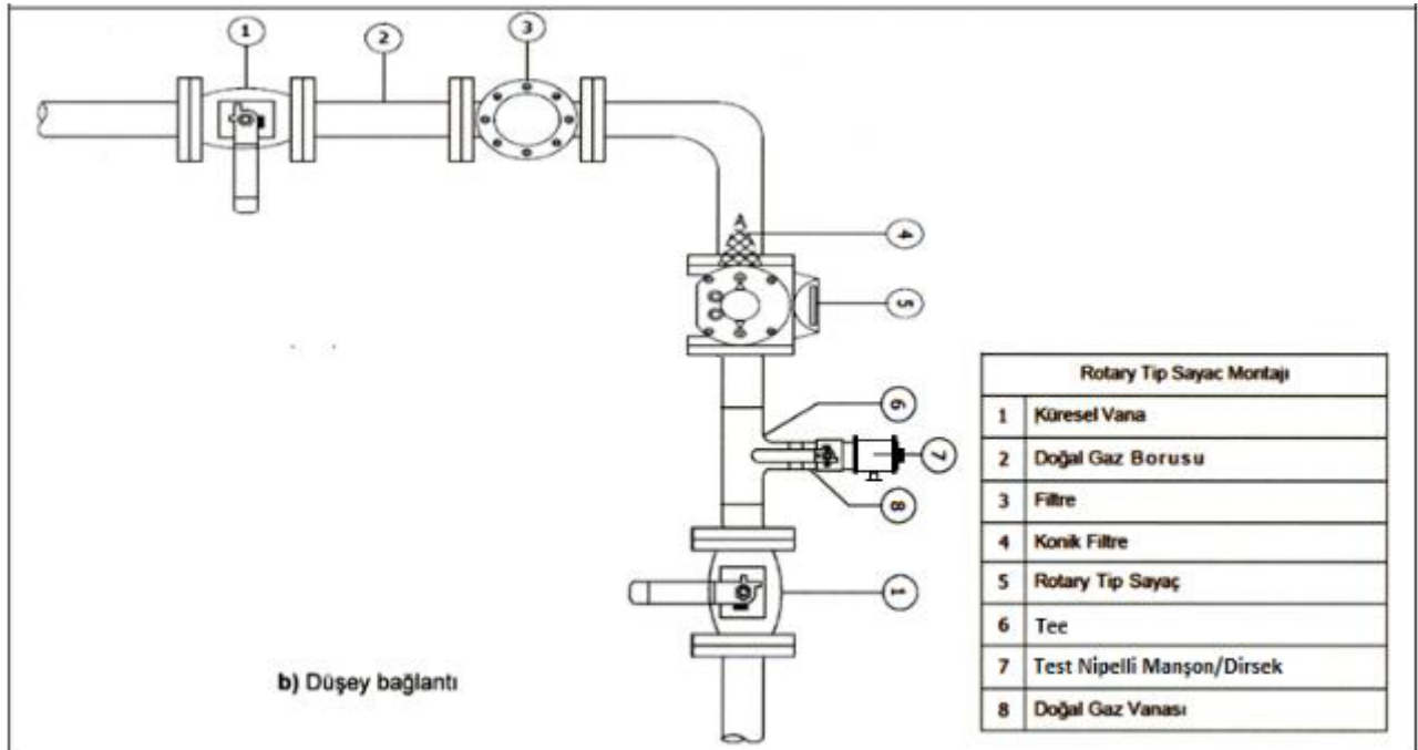
Şekil 16 — Rotary sayaçlara ait bağlantı detayı
