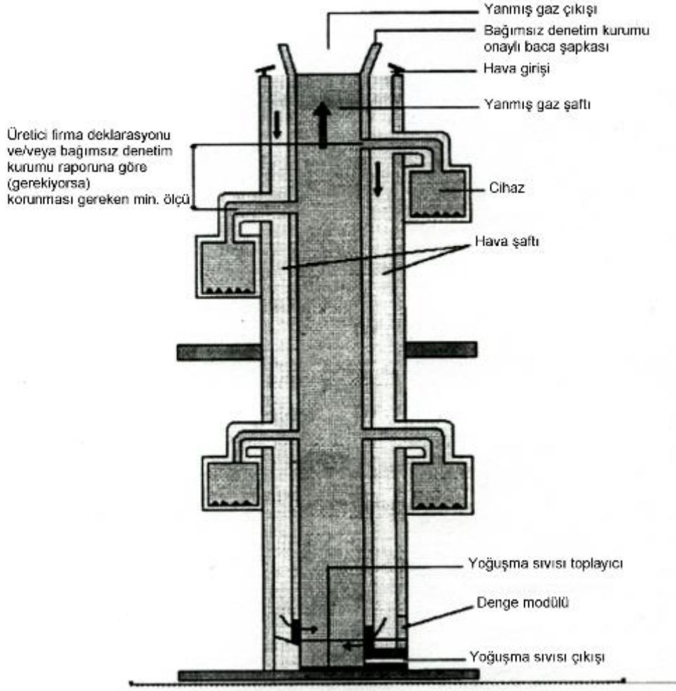
Şekil 29 - Hava-atık gaz baca sistemleri
