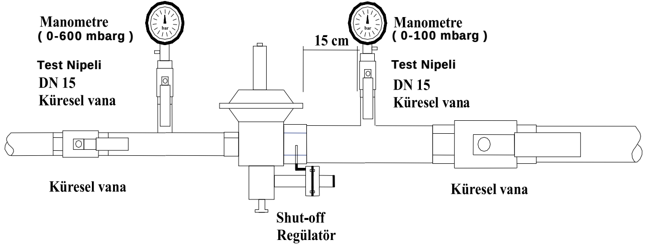
Şekil 13 Shut-Off Regülatör
