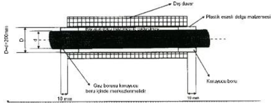
Şekil 9 Duvar Geçişi
